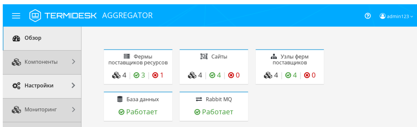
Рисунок 2 – Окно функции «Обзор» в графическом интерфейсе управления Агрегатора
