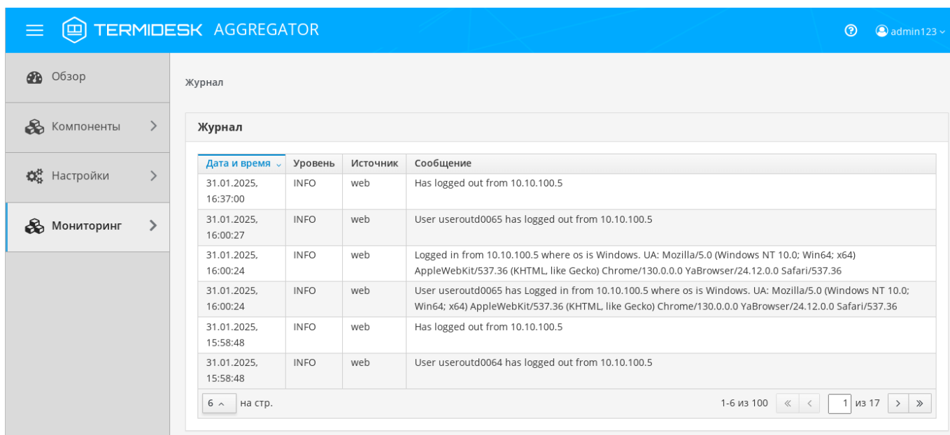
Рисунок 7 – Отображение общего журнала событий
