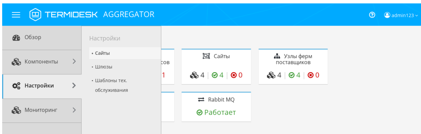
Рисунок 4 – Окно функции «Настройки» в графическом интерфейсе управления Агрегатора
