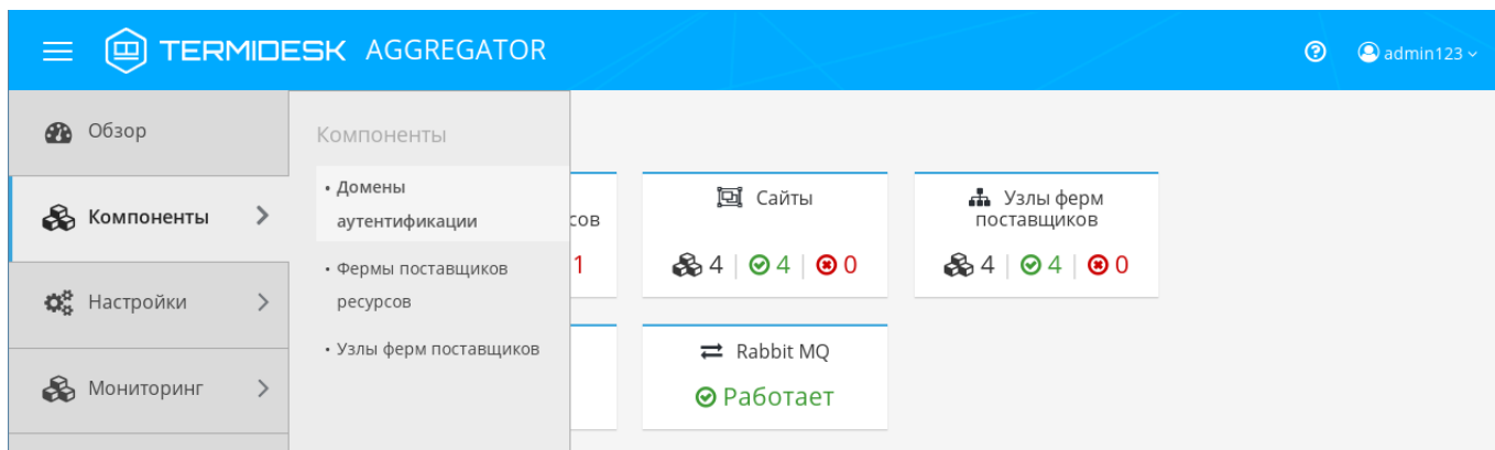
Рисунок 3 – Окно функции «Компоненты» в графическом интерфейсе управления Агрегатора
